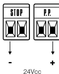
Схема подключения питания фотоэлементов к приводам Spin
