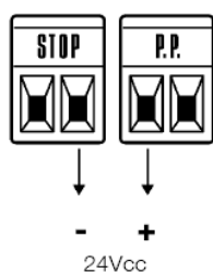
Схема подключения питания фотоэлементов к приводам Robus
