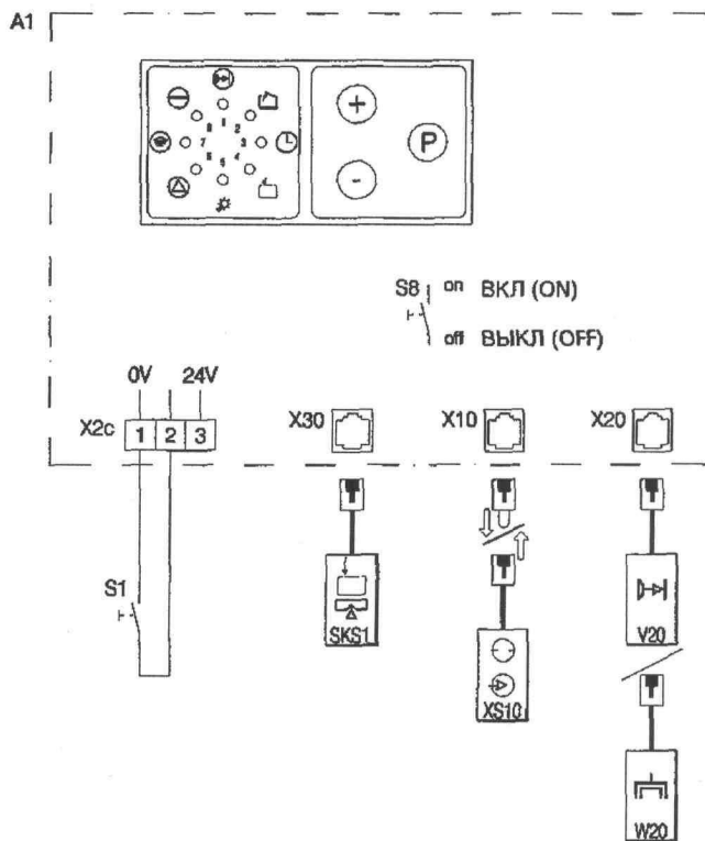
Рис. 12: Элементы системы управления C14 / C15
